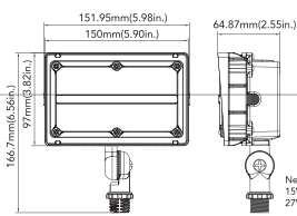
15W&27W(Knuckle Mount)
