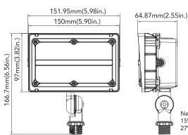
15W&27W(Knuckle Mount)
